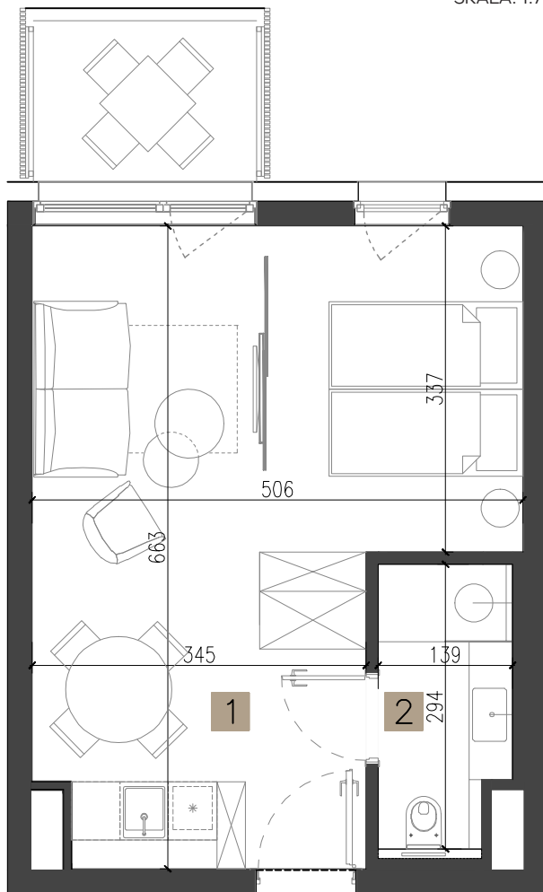
RZUT APARTAMENTU
